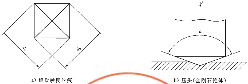
图 1 试验原理
